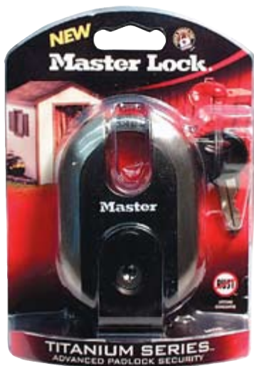
187XD
